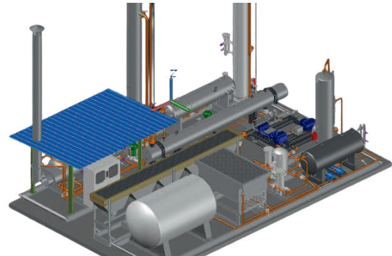
PLANTA PARA ENDULZAMIENTO DE GAS
